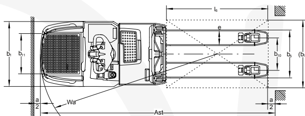
Plataforma de pie fija
